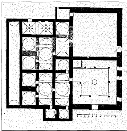
Ibrâhim Paşa Hamamı'nın planı (Glück, şekil 105)
